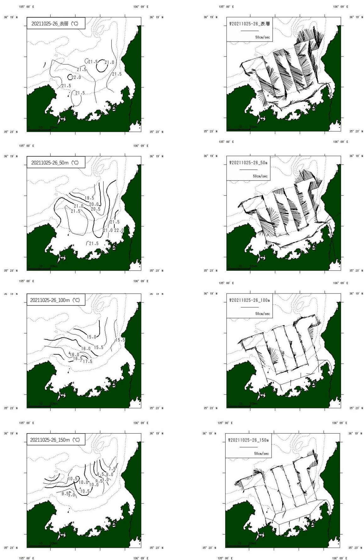
図 若狭湾海域水温および流向・流速水平分布 (令和3年10月25日～26日)
