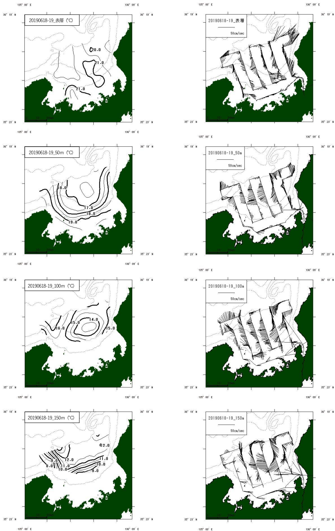
図 若狭湾海域水温および流向・流速水平分布（令和元年6月18日～19日）
