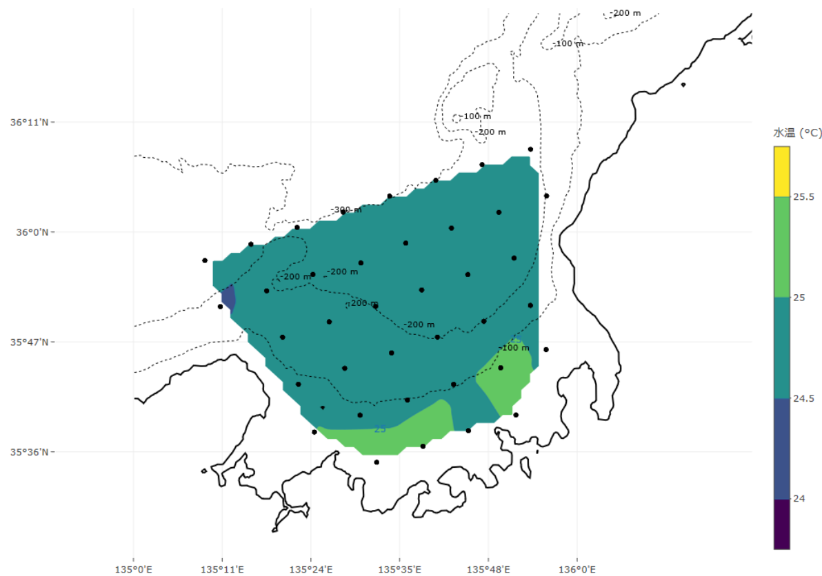
5 m水温
