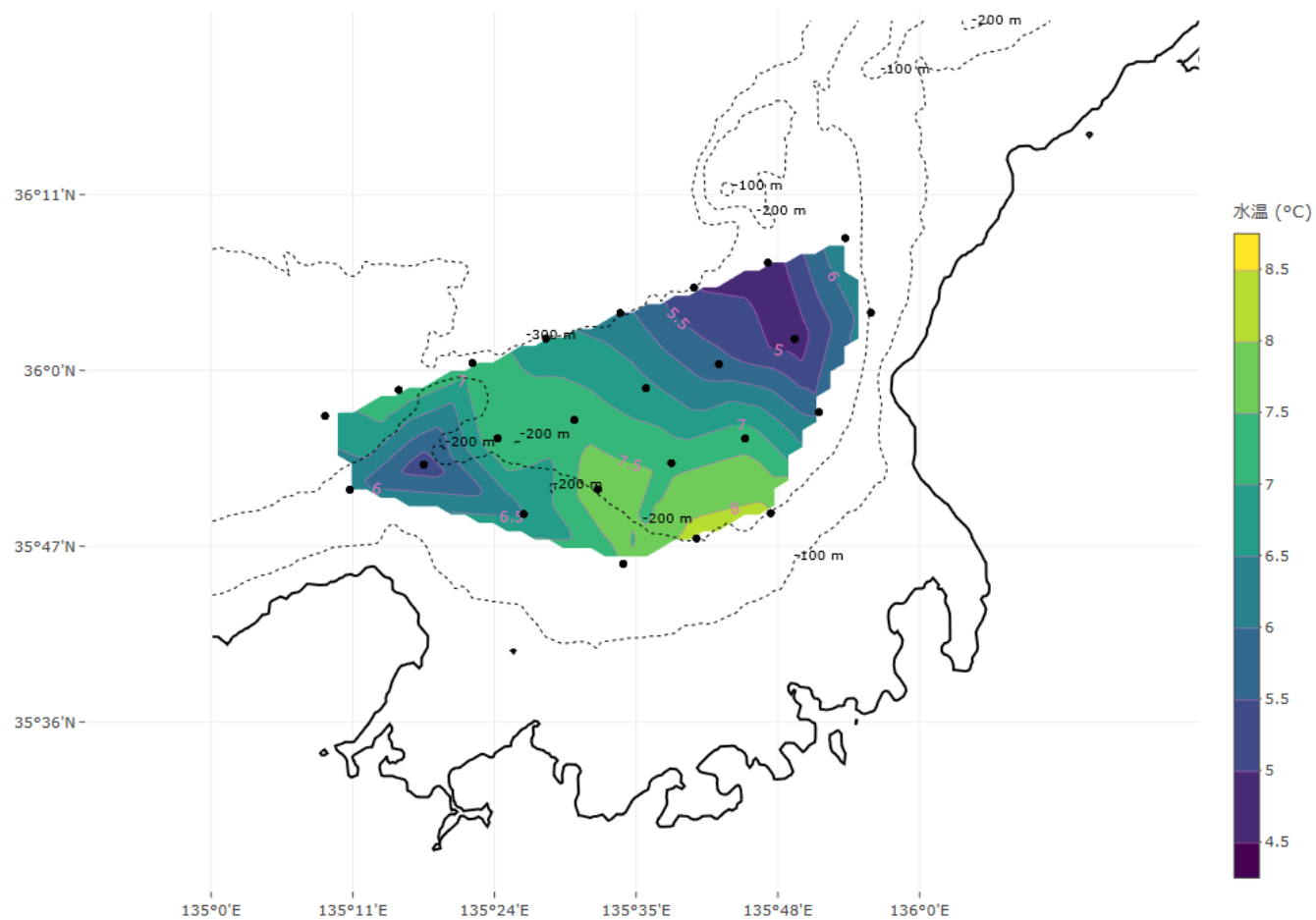
150m 水温
