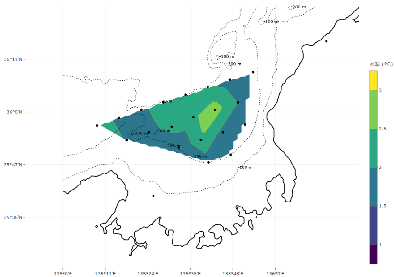
200m 水温
