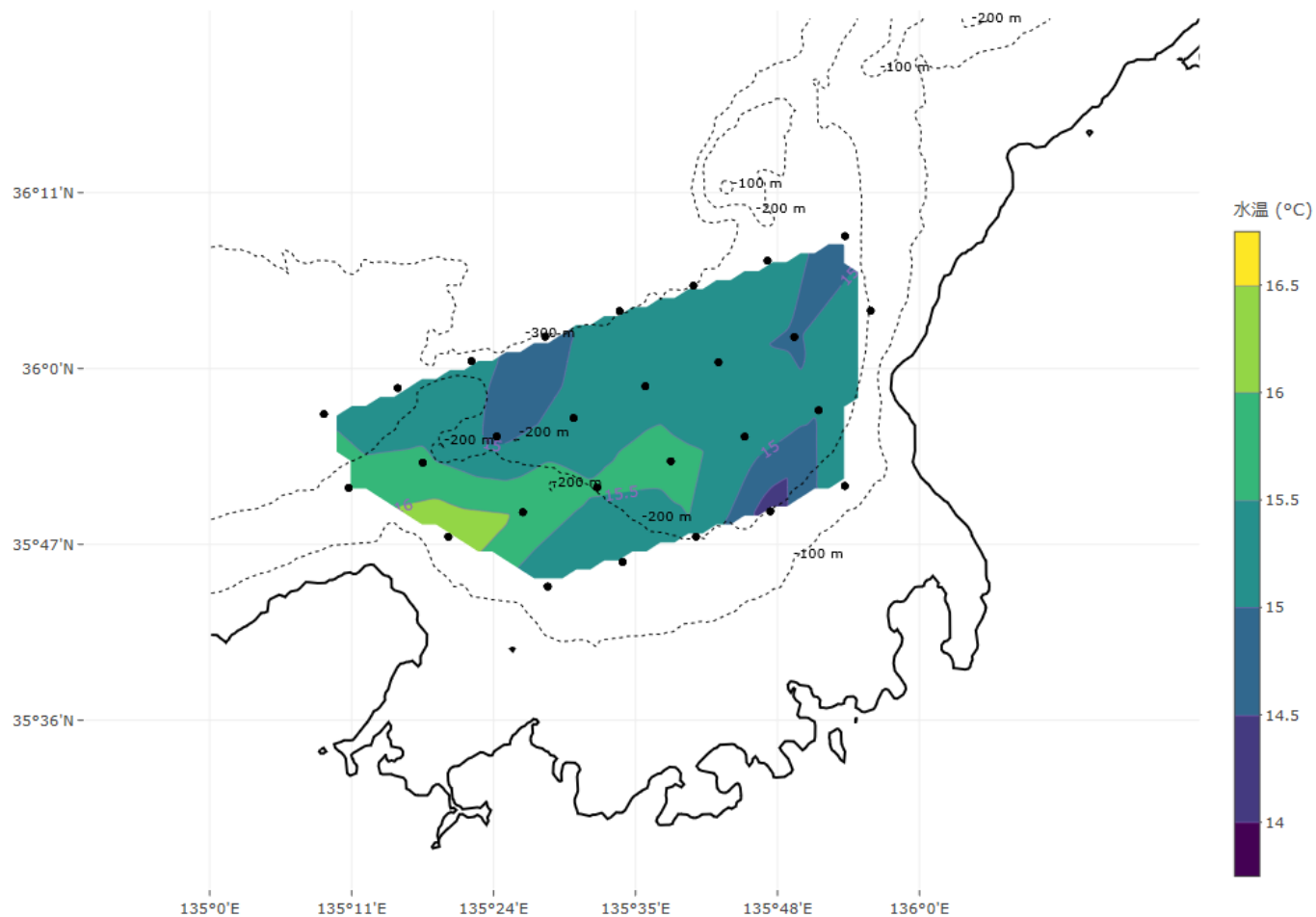
150m 水温
