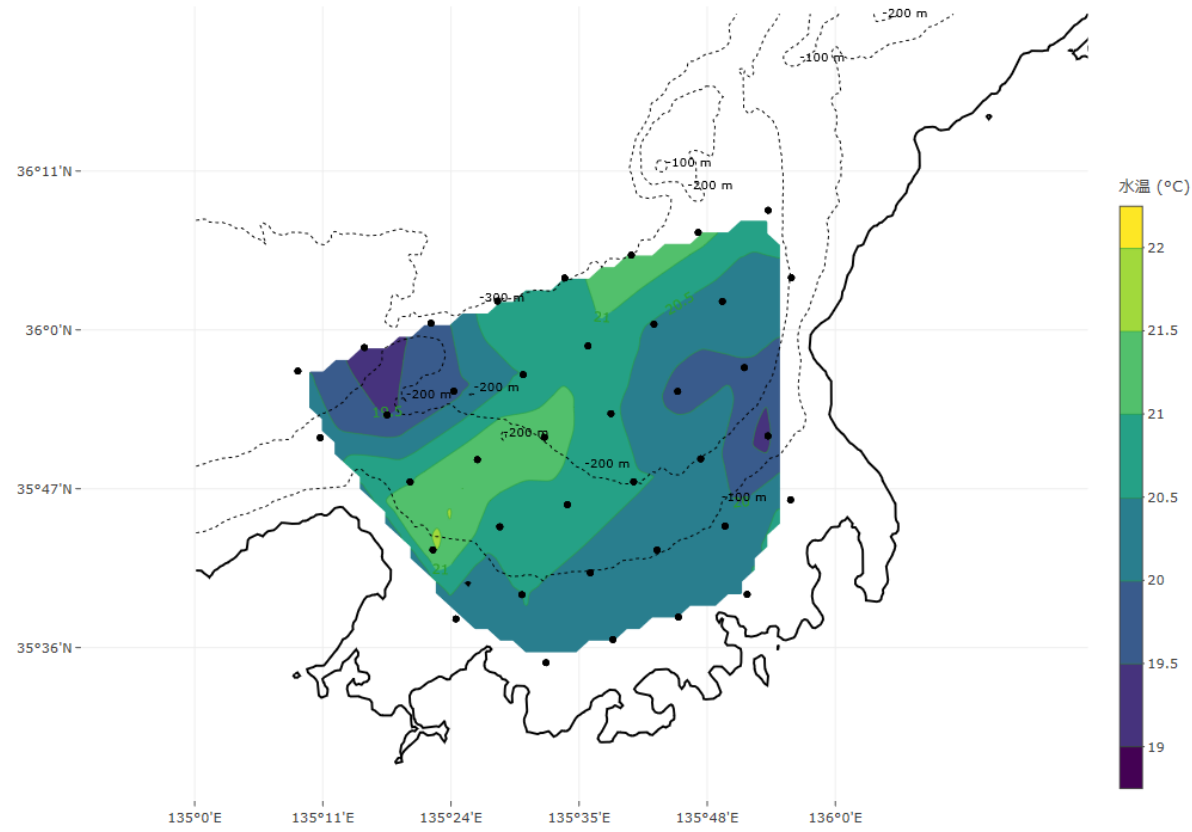
100 m 水温
