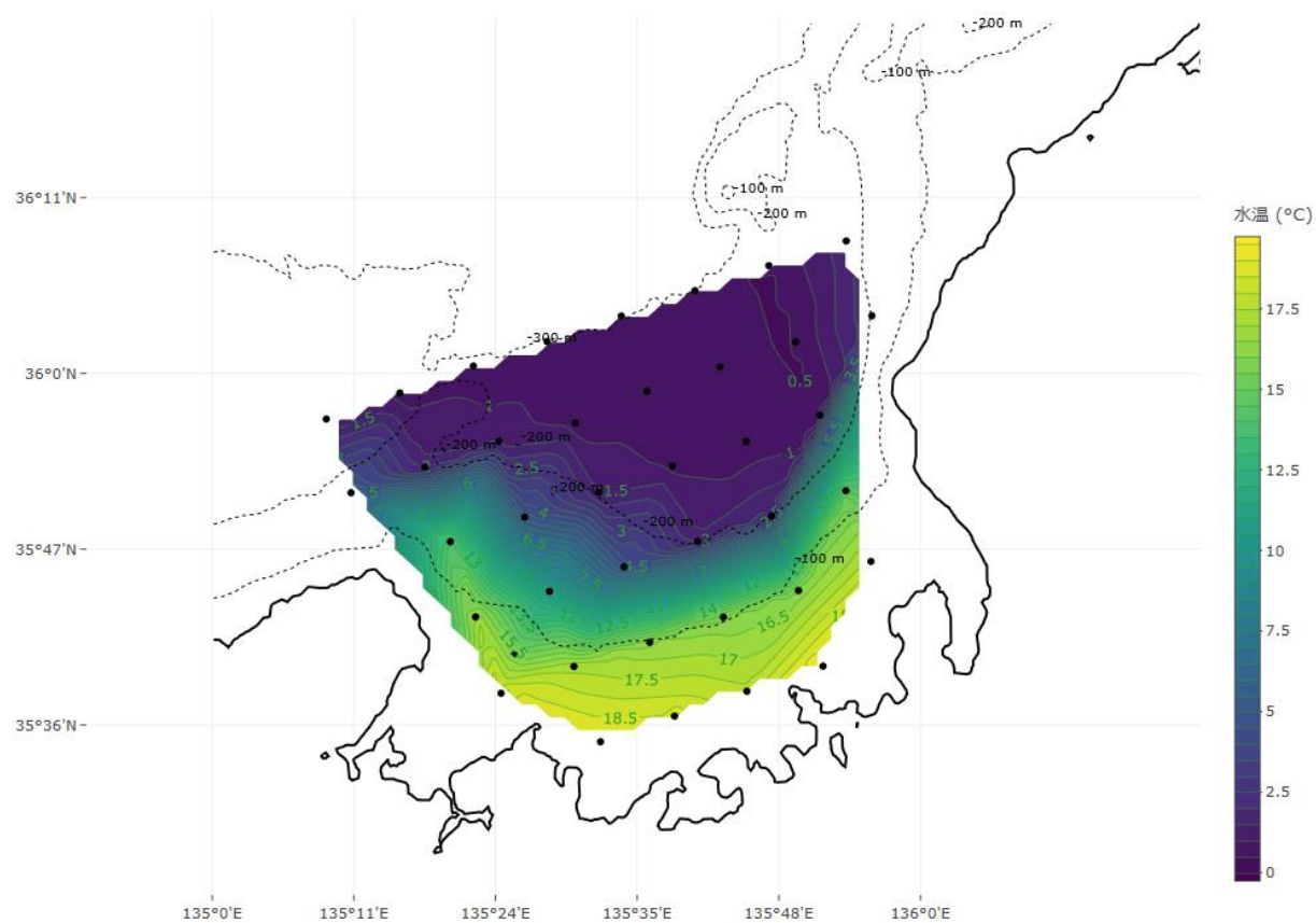
底層水温
