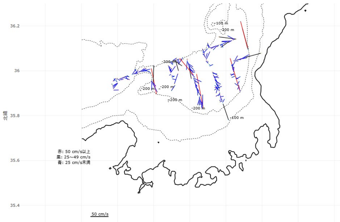
200 m 付近流速
