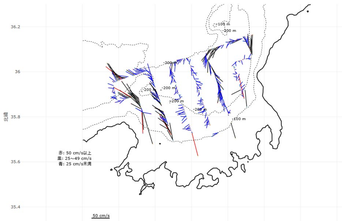
100 m 付近流速
