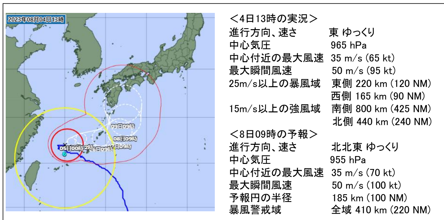
図 2. 気象庁による台風情報
