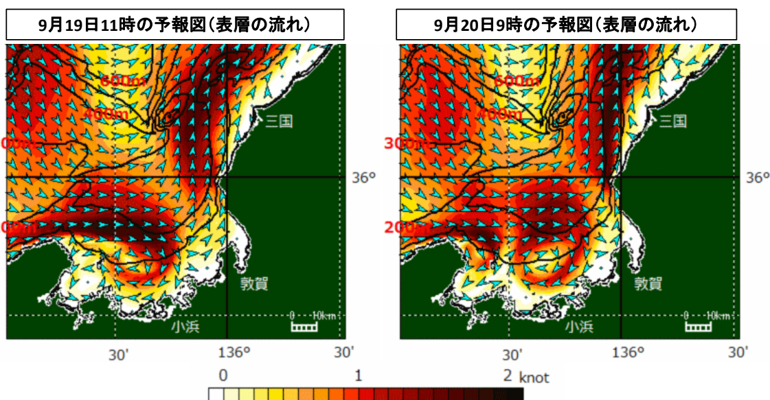
図1. 流況予報図
