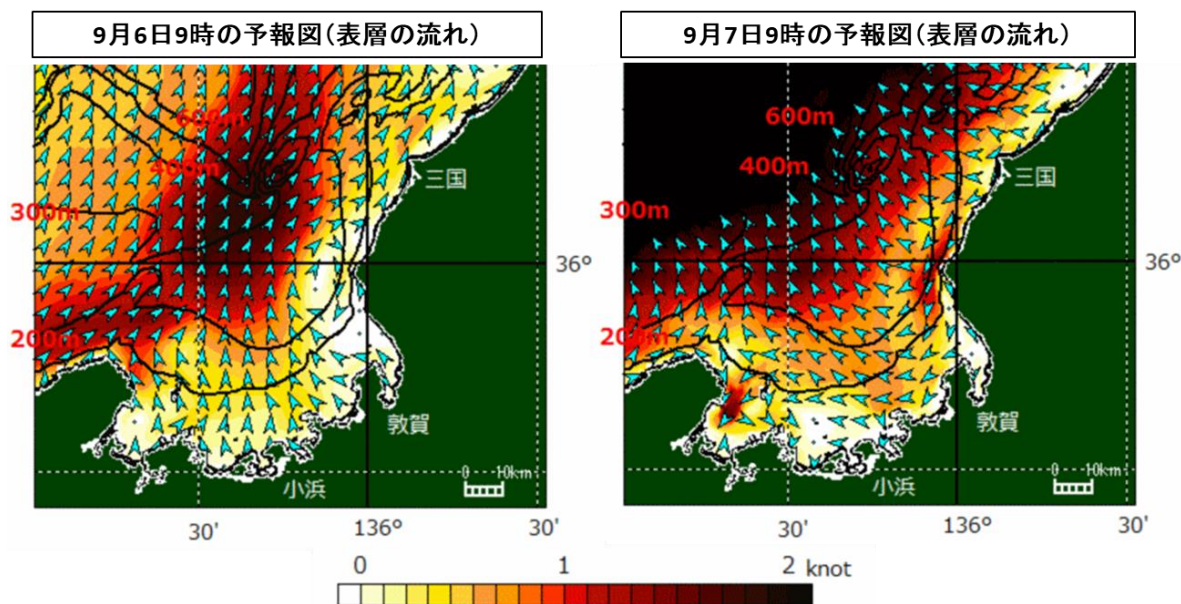
図1. 流況予報図
