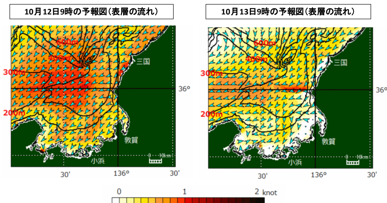
図1. 流況予報図
