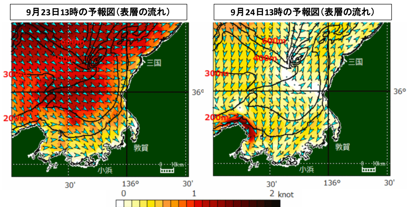
図1. 流況予報図
