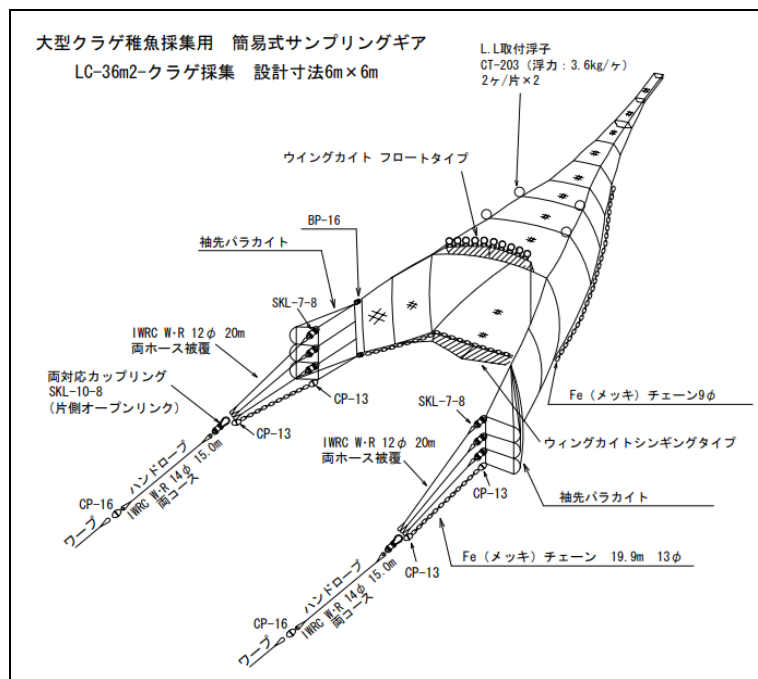
図2 LCネット模式図
