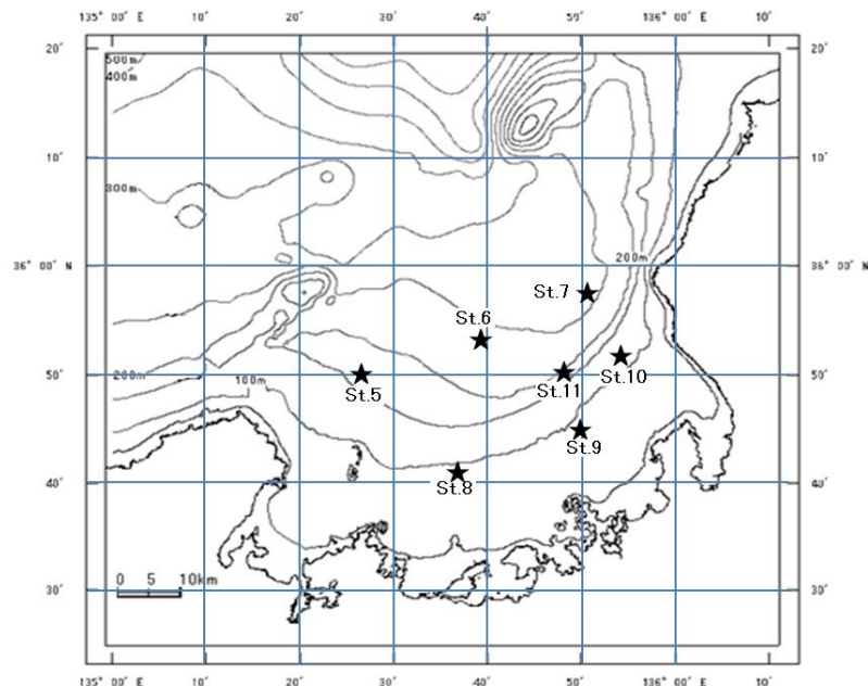
図. 大型クラゲ分布目視調査海域
