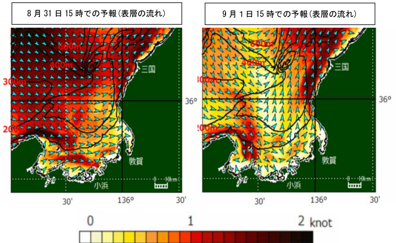
図 3. 流況予報図
