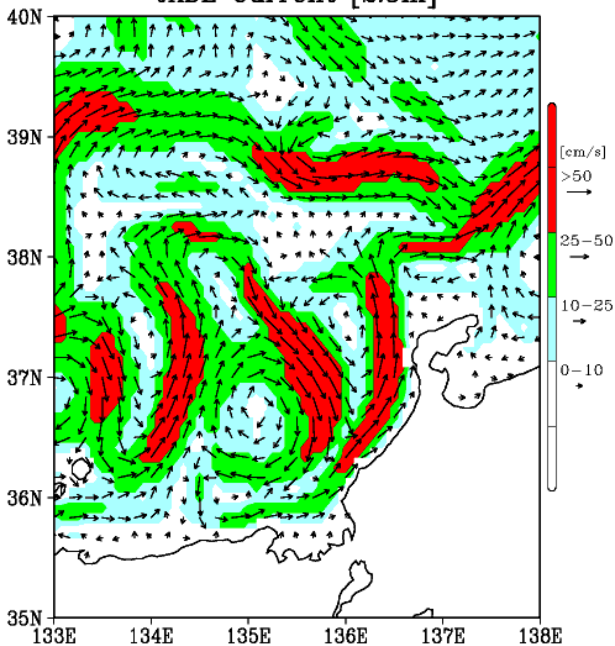
図4. 日本海区水産研究所による流況予測結果
