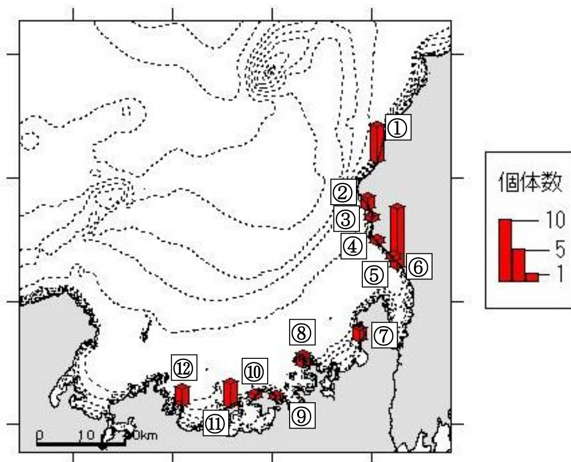
図2. 県内定置網への入網状況（8月26日～9月9日）
