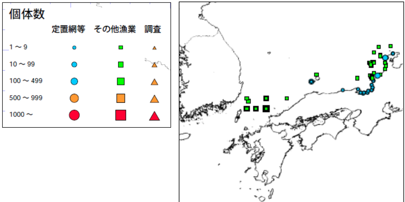
図3 日本海および東シナ海における大型クラゲの分布状況（9月9日時点）
