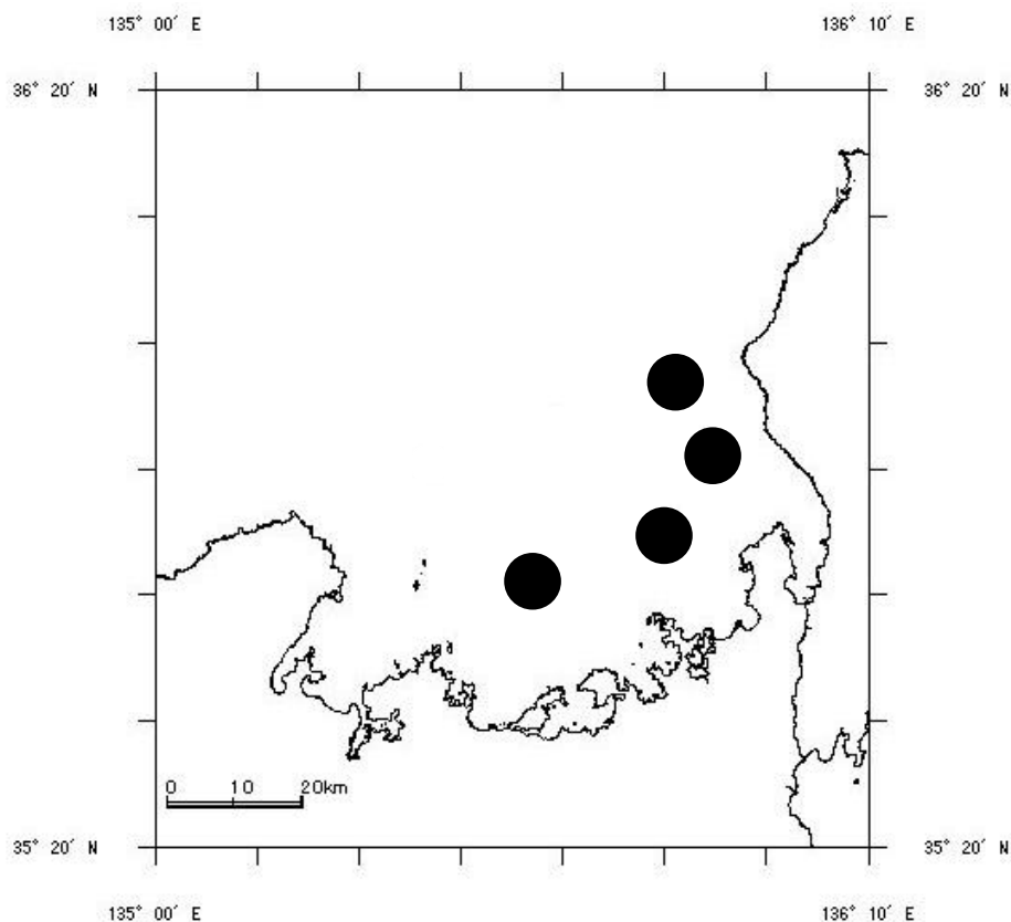
図 1. ネットおよび目視調査定点
